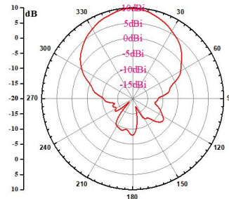
E-plane
