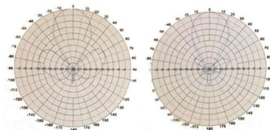
H-plane
